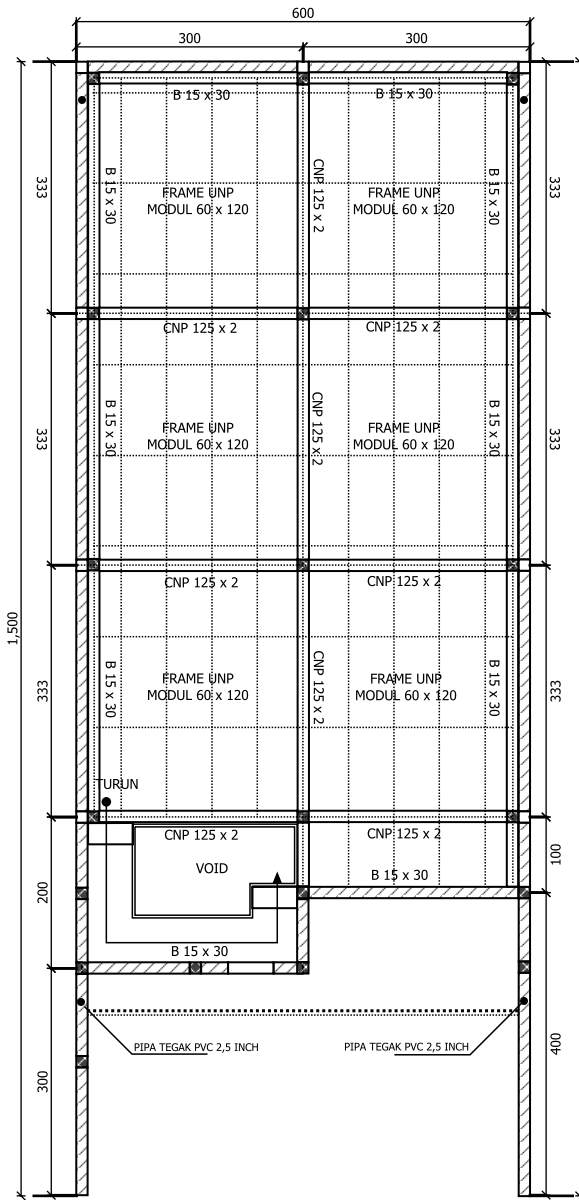
DENAH BALOK LANTAI 2 SKALA 1 : 100
