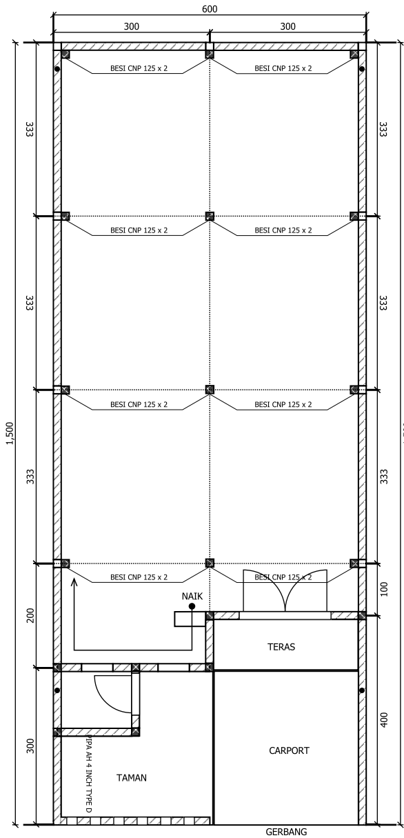
DENAH KOLOM LANTAI 1 SKALA 1 : 100
