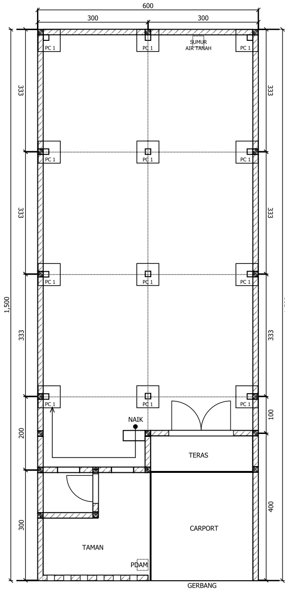
DENAH PONDASI SKALA 1 : 100
