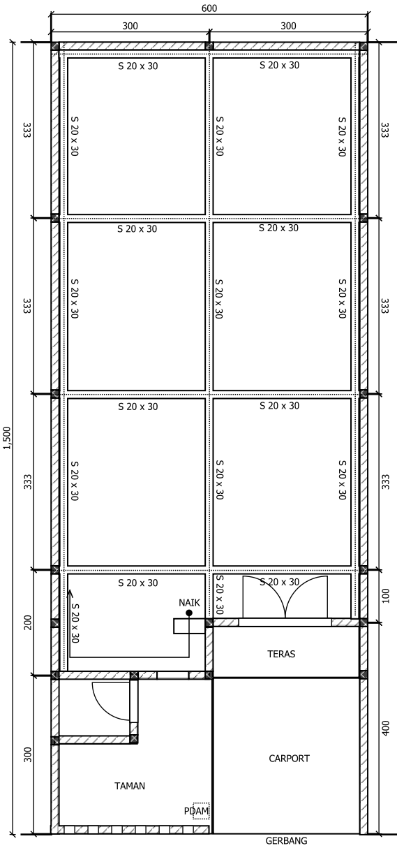
DENAH SLOOF SKALA 1 : 100
