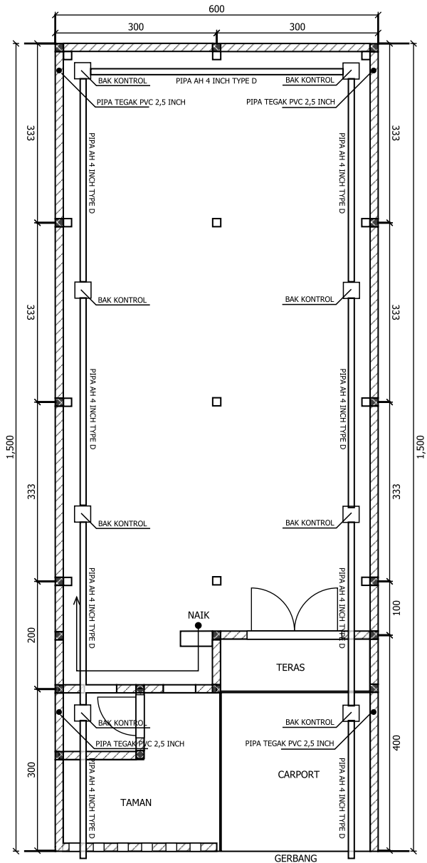
INSTALASI AH/ABK LANTAI 1 SKALA 1 : 100
