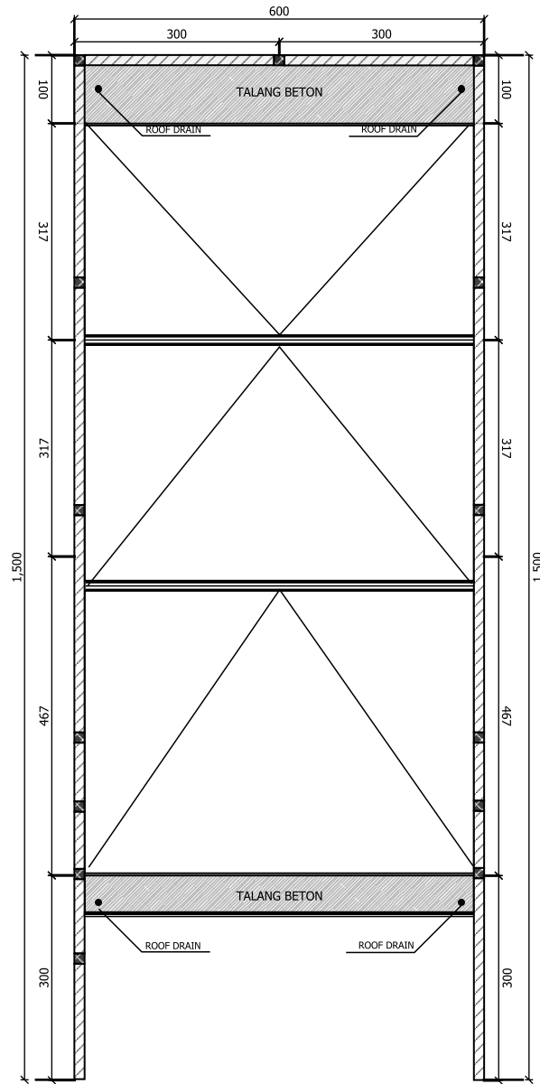
INSTALASI AH ATAP SKALA 1 : 100
