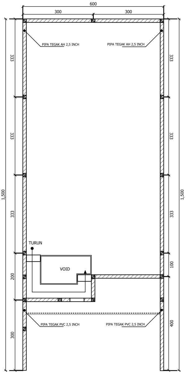
DENAH AH LANTAI 2 SKALA 1 : 100
