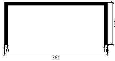
POTONGAN MONKEY BAR SKALA 1 : 75
