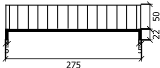
POTONGAN JEMBATAN KESEIMBANGAN SKALA 1 : 75
