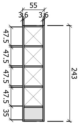
POTONGAN DEPAN RAK SKALA : NTS
