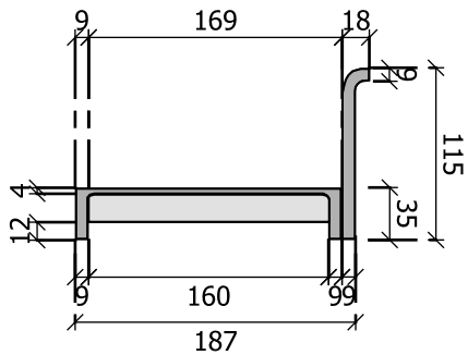
POTONGAN RANJANG C SKALA : NTS
