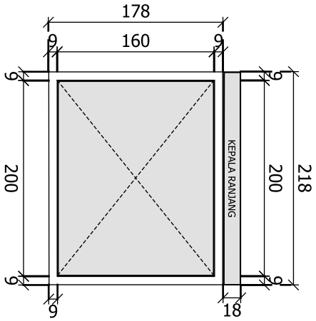
POTONGAN RANJANG A SKALA : NTS
