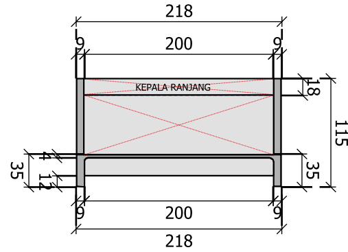
POTONGAN RANJANG B SKALA : NTS
