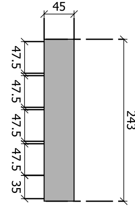
POTONGAN SAMPING RAK SKALA : NTS
