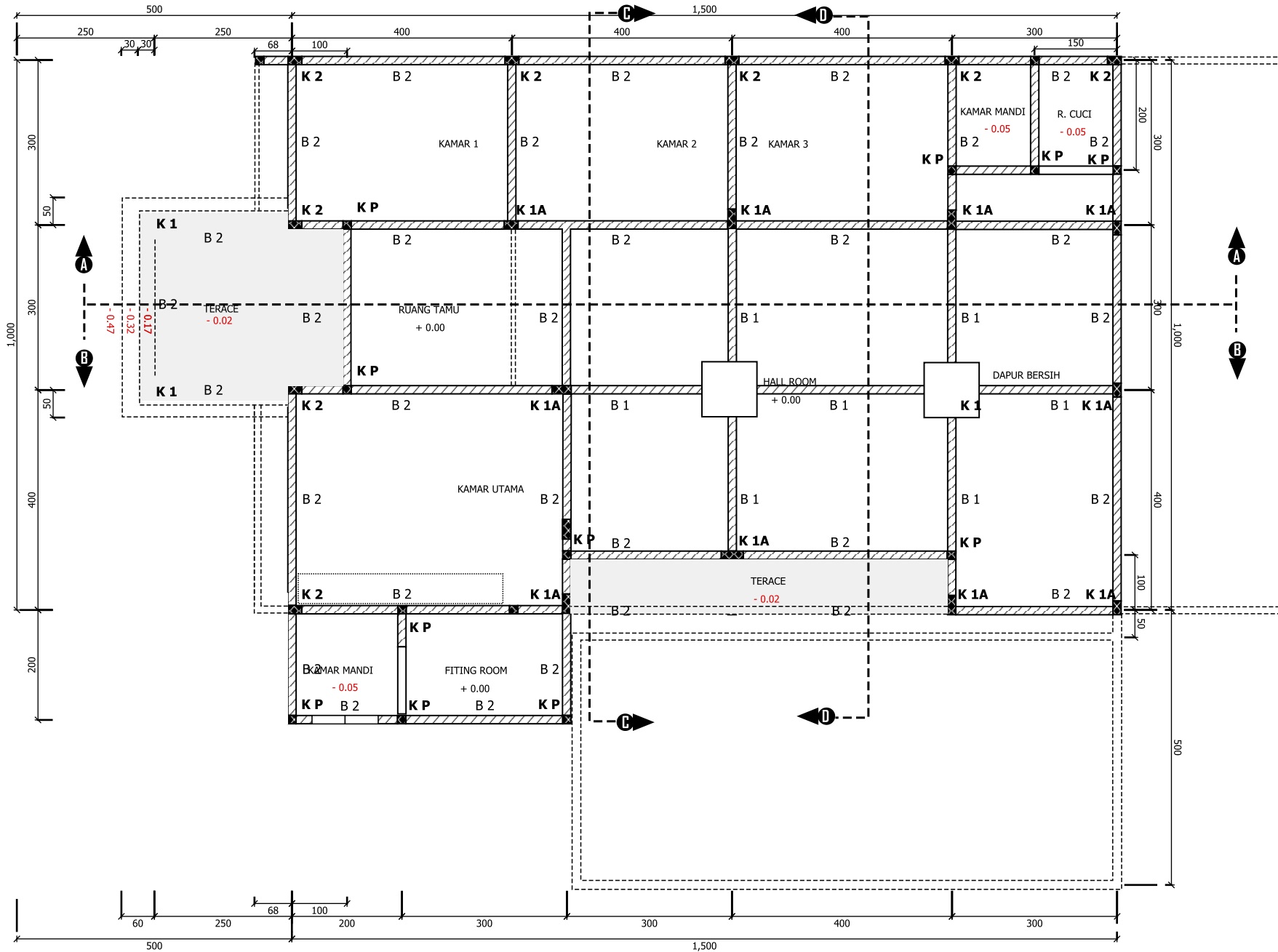
DENAH KOLOM LANTAI 1 SKALA 1 : 100
